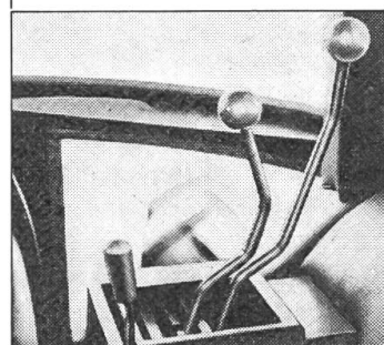
Neue Zwei-Hebel-Schaltung für insgesamt 16 Vorwärts- und 8 Rückwärtsgänge. 8 Gänge lassen sich ohne Kupplung schalten.
