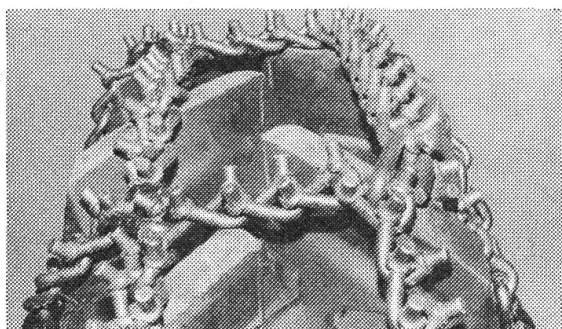
Trygg Stollenkette , Top Qualität zu günstigem Preis. Die beste, bewährte Schneekette, 9 mm ge- härteter Spezialstahl, 2 Stollen pro Kettenglied, ruhig laufend, spurtreu, problemlose Montage.
