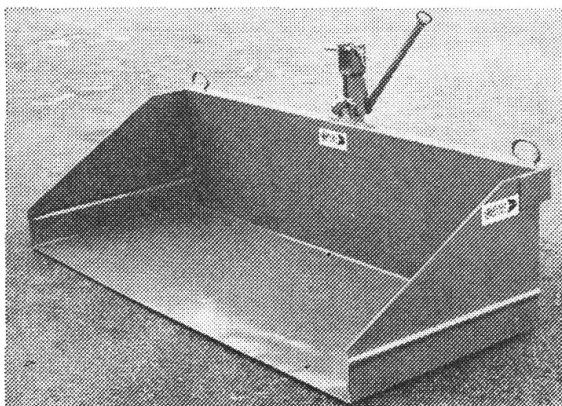
Bärtschi Mehrzweck-Ladeschaufel mit Rollen-Kippvorrichtung, leicht ausklinkbar, sicher, keine Pneubeschädigungen. 3 Grössen, auf Wunsch mit Rückwand-Erhöhung.
