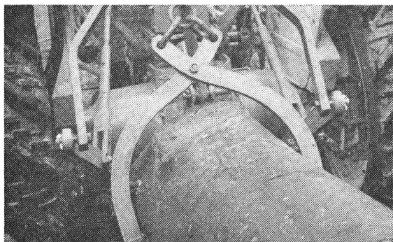
Bärtschi Holzschleppzange für Traktorhydraulik und Seilzug. Kat. I und II. Vielsei- tig, robust, tausendfach bewährt. Auf Wunsch mit Staplerarme, Würgeseile und 3fachem Kettenge- hänge.
