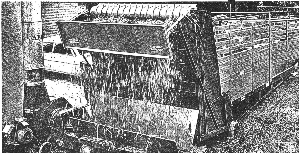
3 Sauggebläse HG 0, HG 1 und HG 8, für Dürrfutter und Welkheu
