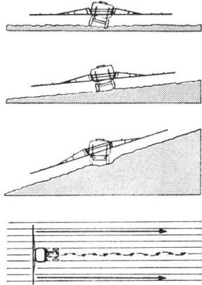
Balkenwippe FISCHER GRAVIMATIC
