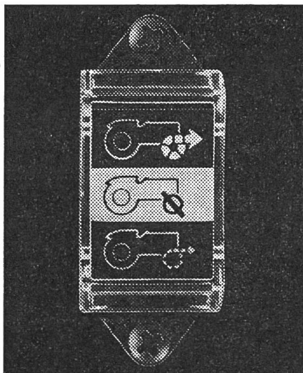
Ein einfacher Kippschalter übernimmt das Zu- und Abschalten des neuen mechanischen Frontantriebes. Ist der Allradantrieb eingeschaltet, leuchtet eine Kontrollampe am Armaturenbrett.
