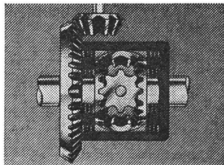
Der vollintegrierte Frontantrieb bezieht seine Kraft direkt aus der Mitte des Getriebes. Das automatische Sperrdifferential verriegelt die Vorderräder, noch bevor ein Rad durchdreht.
