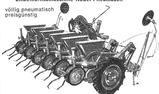
Einzelkornsämaschine Nodet-Pneumaten
