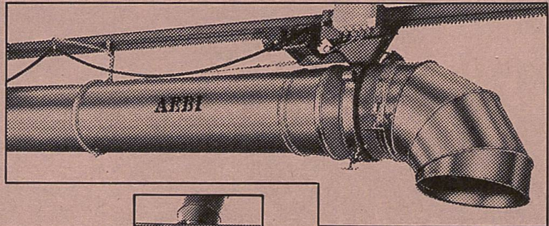
Luft- getriebener Siloverteiler AEROMATIC
