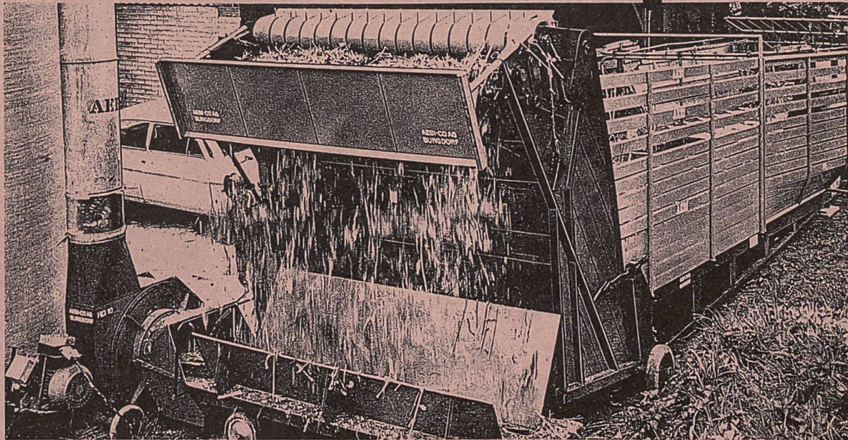
3 Sauggebläse HG0, HG1 und HG8, für Dürffutter und Welkheu
