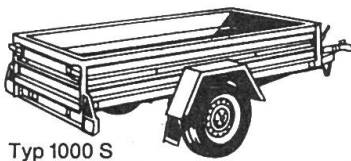
Typ 1000 S mit Kippbrücke 244×122×40 cm Nutzlast 740 kg
