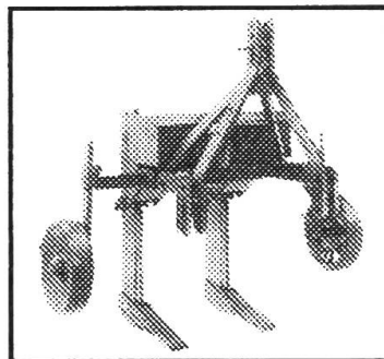
WIPPSCHARLOCKERER
