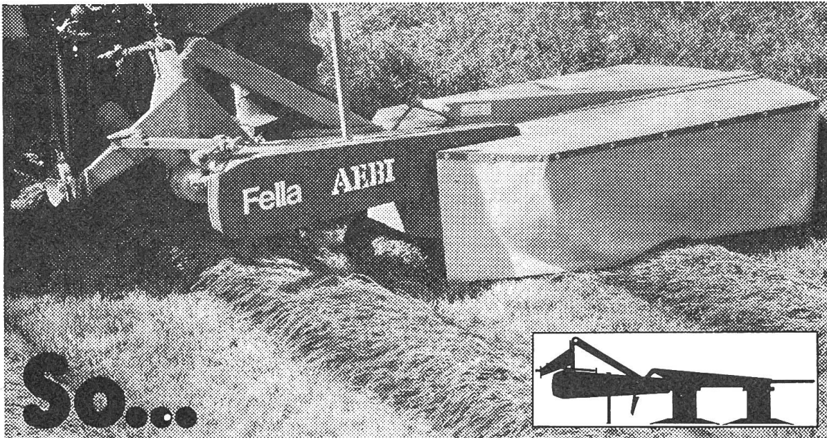
So... Fella Kreiselmäher KM165 und KM190 Arbeitsbreiten 1,65 und 1,90 m. Antrieb über Keilriemen und Kegelradgetriebe im Fettbad. Auflaufsicherung und automatische Transportverriegelung. Messerwechsel mittels Schnellverschlüssen. Bodenanpassung nach oben 30° und nach unten 18°.
