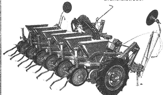
Einzelkornsämaschine NODET-PNEUMASEM mit zentral aufgebautem Granulatstreuer
