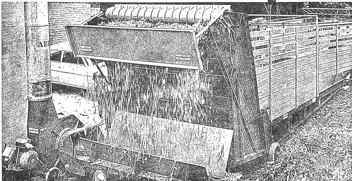
Automatischer Teleskop-Grossflächenverteiler vom Boden aus bedienbar, mit Rückstreu-Vorrichtung, Metalltragschiene ohne Holzbalken
