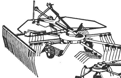
Wirbelschwader
