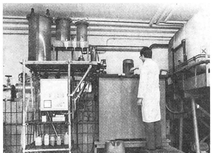
Abb. 1: Teilansicht der vollautomatischen Anlage zur Entgiftung von Härtereiabwässern mit Wasserstoffperoxid in der Degussa-Zweigniederlassung in Hahnau-Wolfgang. (Degussa-Bild)
