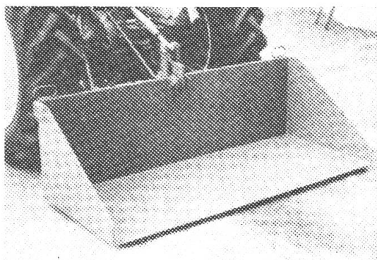
Mehrzweck-Ladeschaufel mit Kippvorrichtung. Für Transport aller Güter, Ausplanieren von Wegen und Strassen und Schneeräumung, 170 und 190 cm.
