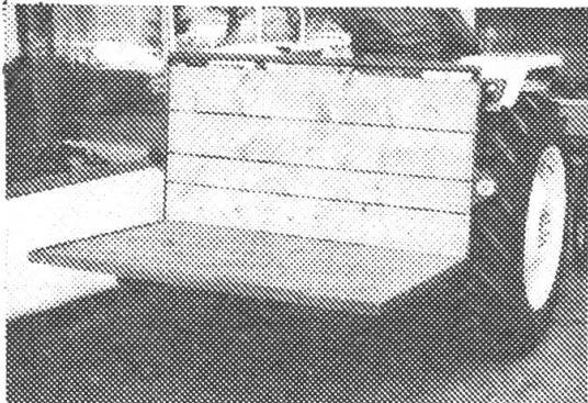
Ladebrücke zu Traktoren , zweckmässig und stark, Ladefläche 140 x 100 cm, Tragkraft 400 kg.
