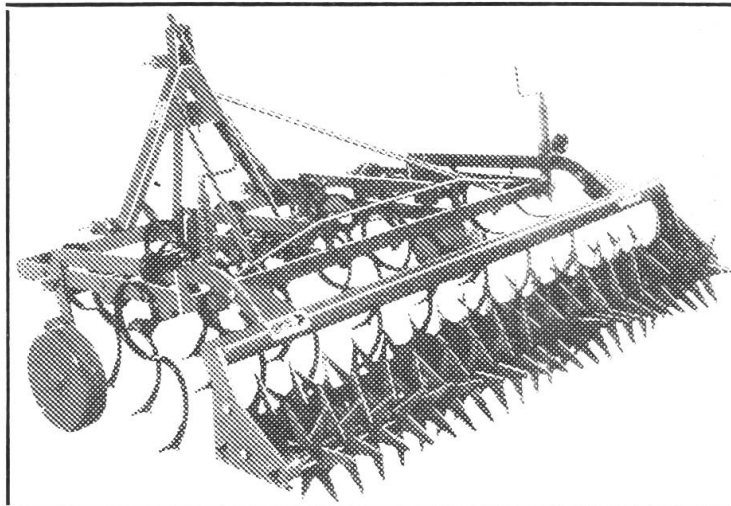
Bärtschi-Federzahnegge mit Doppelsternkrümmer
