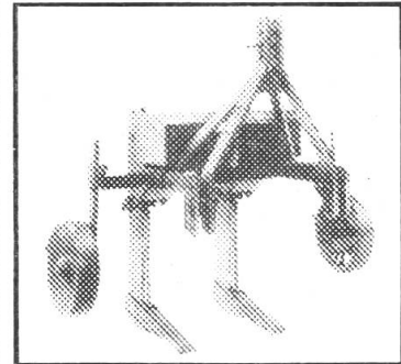
WIPPSCHARLOCKERER
