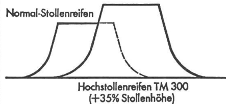
Aufstandsfläche TM 300
