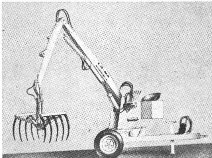
LO-MA-Mistladekran, 3 Punkt, mit hydr. Abstützung Fr. 5400.-, gerogen Fr. 5500.-
