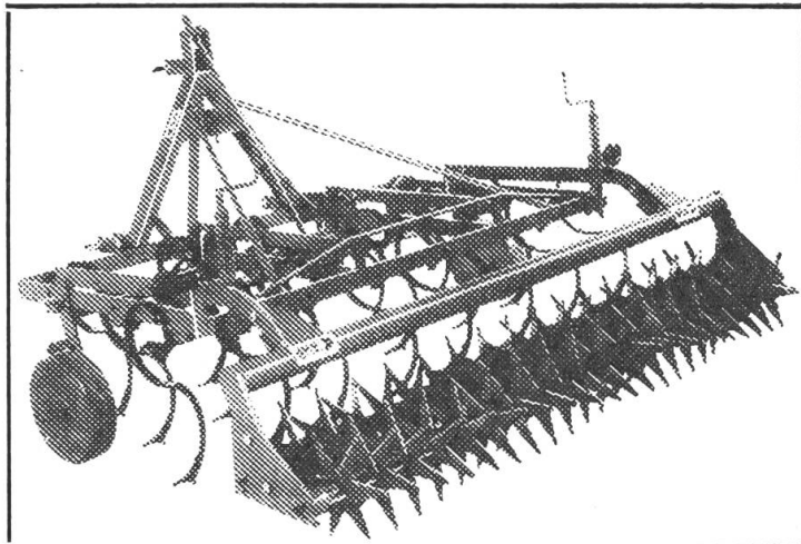
Bärtschi-Federzahnegge mit Doppelsternkrümmer
