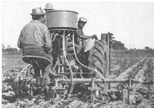
ACCORD Hackgeräte, Reihenfräse OMPI. vielseitig kombinierbar, 2–7-reihig, mit Düngersteuer Roll-Culi, 2–6-reihig.
