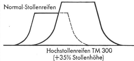
Aufstandsfläche TM 300
