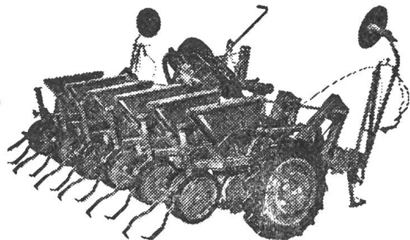
NODET-Einzelkornsämaschinen für Mais, Bohnen, Gemüse usw.
