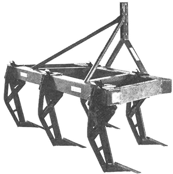
Tiefgrubber, verschiedene Chassis und Zinken
