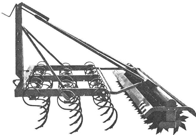
Kultureggen mit 2-Walzen- oder Spatenkrümmer
