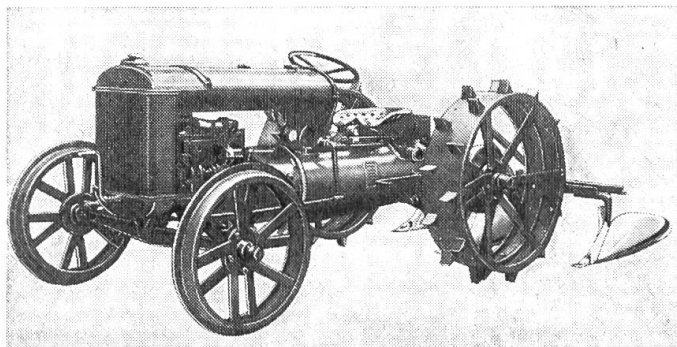
Abb. 3: Der «Black Traktor», Prototyp-Traktor mit Ferguson-System aus dem Jahre 1933.
