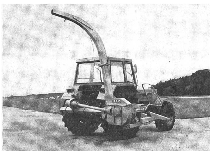
Abb. 1: Anbau-Maishäcksler Claas Jaguar 30 mit senkrecht stehenden Einzugsrollen und senkrechter Messertrommel.
