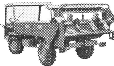
Aufbaumistzetter 2,5 und 3 t
