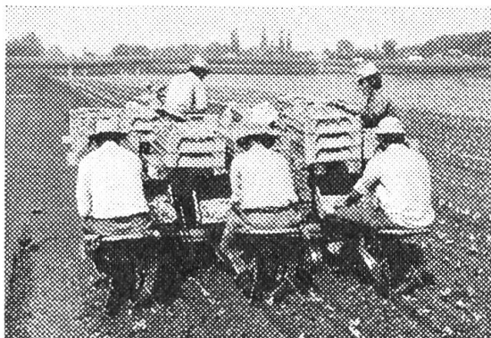
ACCORD Pflanzensetzmaschine, 2–7-reihig, für Gemüse, Tomaten, Tabak, Rosen, Erdbeeren, Forstbäum- chen usw., für Setzlinge und Topfballen.
