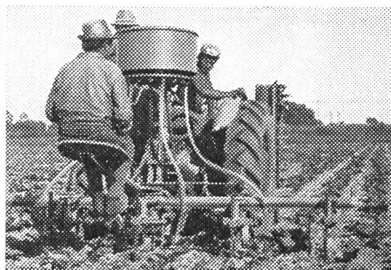
ACCORD Hackgeräte, vielseitig kombinierbar, 2–7-reihig, mit Düngersteuer Roll-Culi, 2–6-reihig. Reihenfräse OMPI.
