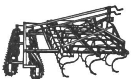
MÖLLER Kultureggen mit Ein- oder Zweiwalzen-Krümler
