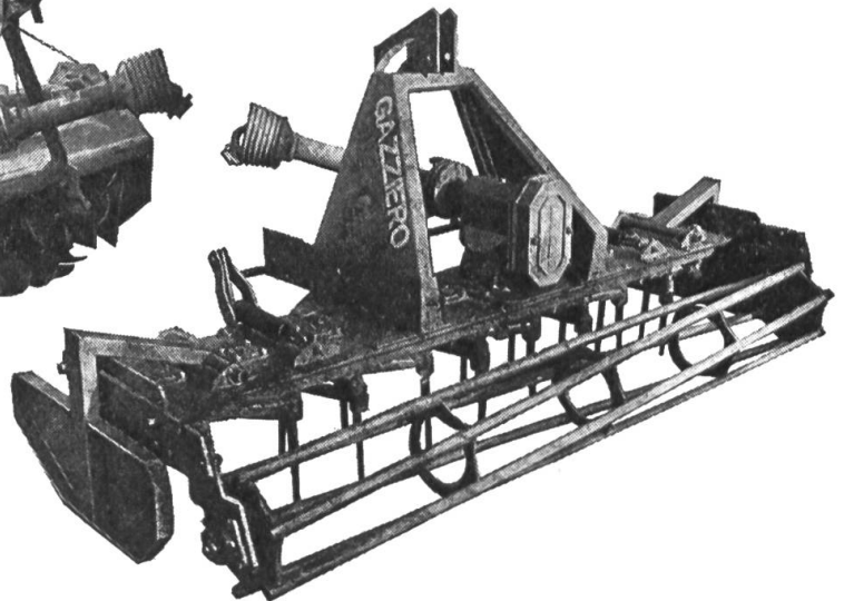
Gazziero-Kreiseleggen
