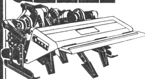
4-Gang-Getriebe. Breiten 20-40 cm. (Für 2- oder 3- von 90-225 cm. Auf Wunsch Punkt). Keine Furchen und mit hydr. Stockräumer. keine Bodenverdichtungen Variable Arbeitstiefen von mehr!
