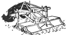
WEICHEL-Tiefengrubber mit Rotor-Egge
