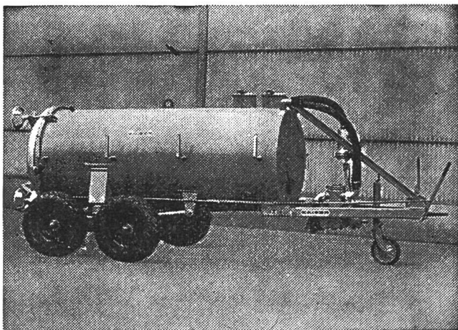
NEU: Gummigefederte Pendelachse ab 4000 Liter Das Fass der Zukunft!
