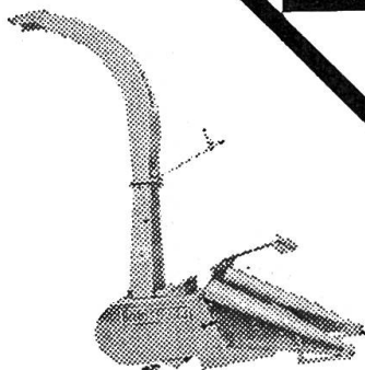
Maishäcksler Hagedorn , dank schnellaufender Trommel mit 9 Messern 25—30t/h, Exakt- schnitt 4,5 mm, Leistungs- bedarf 30—60 PS, Ge- schwindigkeit 5—8 km/h
