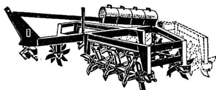
Spatenkrümmer, 2- oder 3-reihig, mit 2, 4 oder 6 Walzen, Arbeitsbreiten von 1,67 bis 2,60 m
