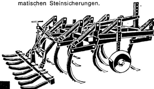
Grubber mit 7, 9, 11, 13 oder 15 starren oder abgefederten Zinken, Arbeitsbreiten von 175 cm bis 360 cm, Rahmenhöhe bis 77 cm.
