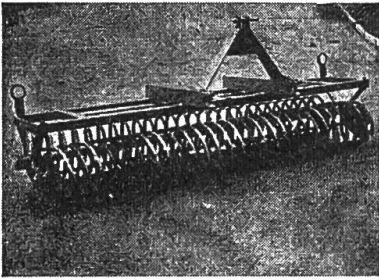
Ringelwalze
