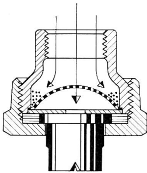
Präzisionsdüse 110° mit Selbst- reiniger
