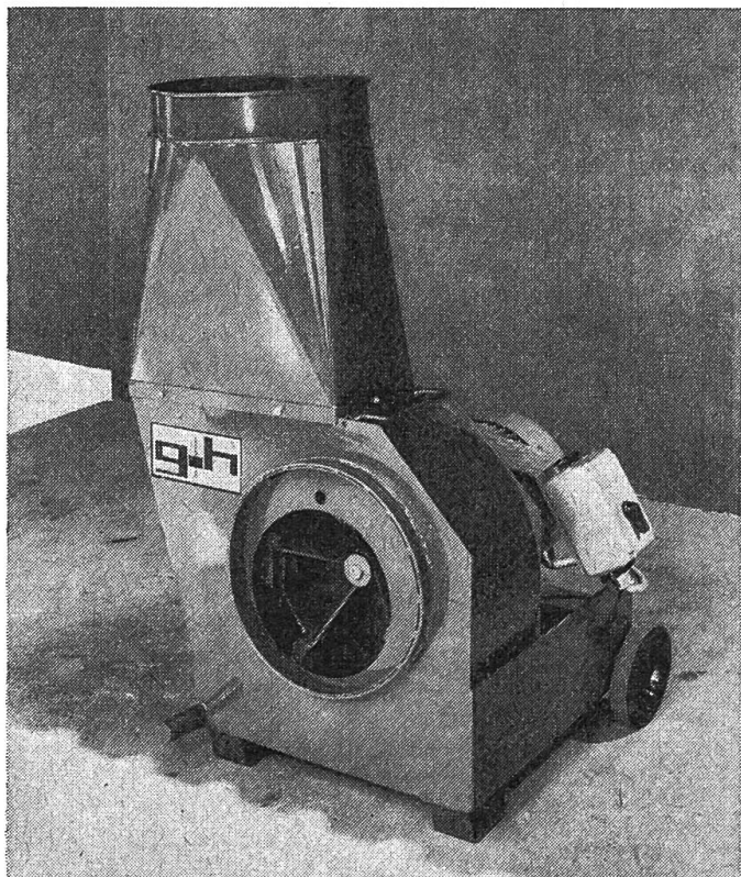
G+H Uni Mill mit Elektromotor
