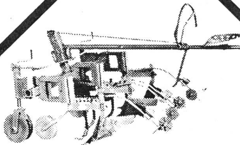
Vielfachgeräte Müller , hier als Hackgerät. Sehr robuste Ganzstahl-Konstruktion, Baukastensystem. Auch für Pferdezug lieferbar.
