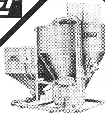
SKJOLD-PICCOLO Mahl-/Mischanlage mit unbegrenzten Möglichkeiten; Zeituhr, Abschaltautomatik usw., fertig verdrahtet, Kabel nach Wunsch. Seit Jahren ein Preisschlager!
