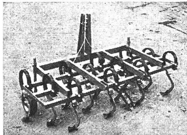
Grubber/Federzahnegge
