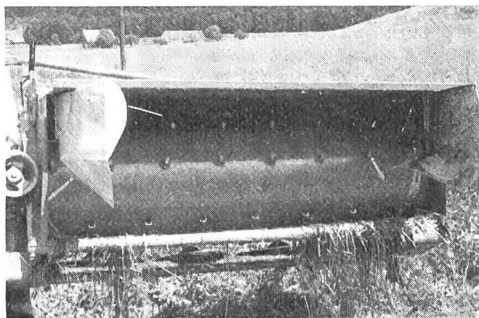
Kreiselmäher mit Aufbereitungstrommel.
