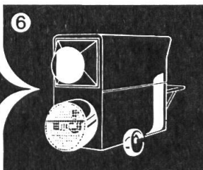
LICO-Heizkessel für Warm-Heubelüftung
