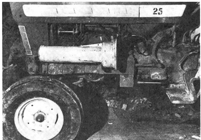
Abb. 2: So wird der Abgasverdünner am Traktor angeordnet.
