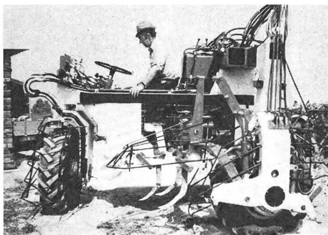
Abb. 1: Seitenansicht des «Hydro-Storch» (Werkbild: A. Rosentreter).
