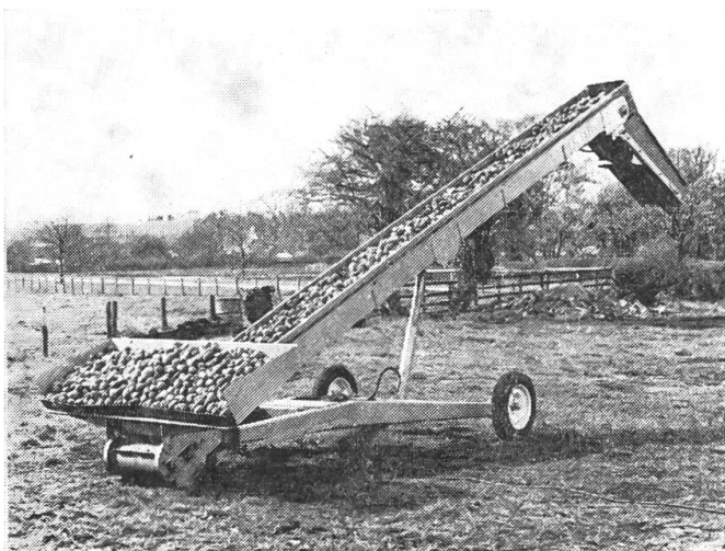
Die Kartoffel-Beförderungsanlage mit endlosem Gummi-förderband, das sich wahlweise mit Elektro- oder Verbrennungsmotoren treiben lässt.
