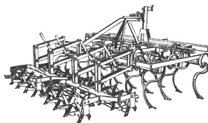
Federzinken-Kultivator mit Krümmler oder Nach- egge
