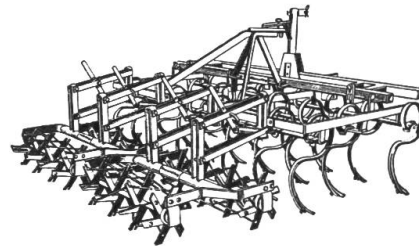
Federzinken-Kultivator mit Krümmer oder Nach- egge
