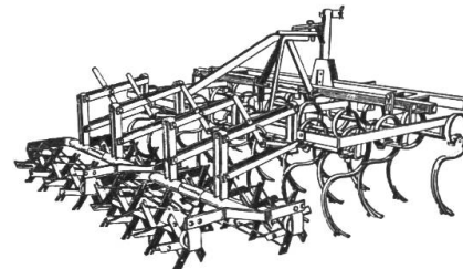
Federzinken-Kultivator mit Krümler oder Nach- egge
