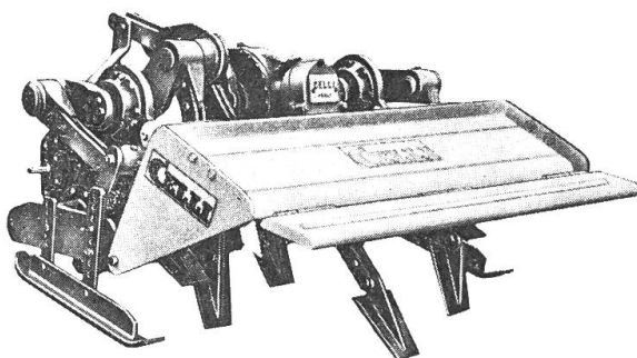
Spatenmaschinen 90–260 cm Arbeitsbreite bis 30 cm Arbeitstiefe für die neuzeitliche Bodenbearbeitung
