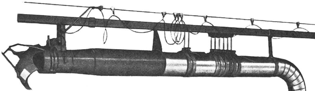
Heuverteileranlage bis 30 m Streubereich (Länge)
