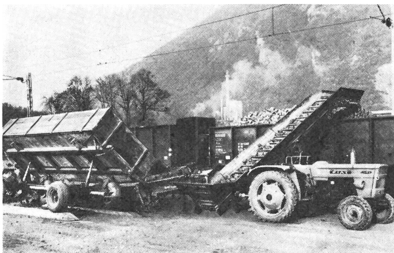
Verladeanlage für Zuckerrüben (Fa. Kunz, Burgdorf).
