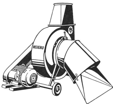
Typ SG III mit Anbaumotor
