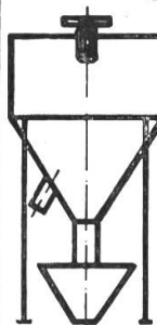
Lager-Silos
