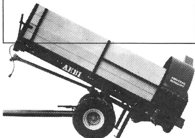
Miststreuer. Leichter Wechsel der Aufbaugeräte
