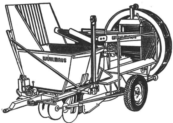
Vollernter-Bunkermaschine
