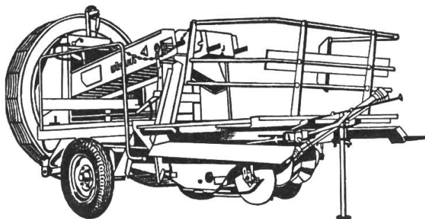
Vollernter-Absackmaschine
