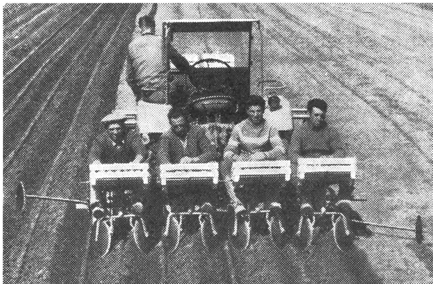
4-reihig Kartoffelhacken mit «Müller»-Patent-Setzautomaten
